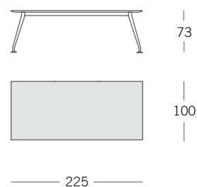
Tavoli meeting piano rivestito o legno Upholstered or wooden meeting tables Tables de reunion avec plateau revetu or en bois
