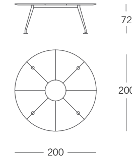
Tavoli meeting piano rivestito Upholstered meeting tables Tables de reunion avec plateau revetu
