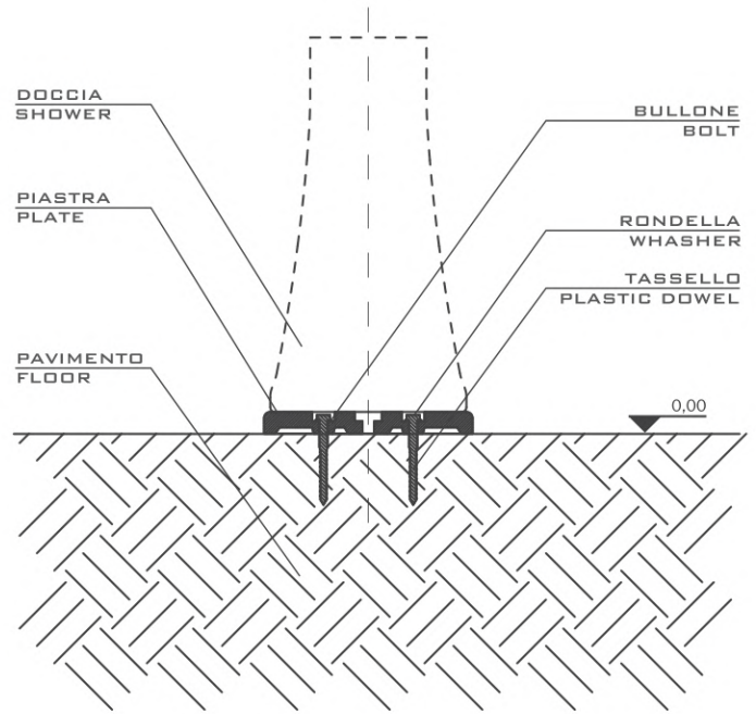
MONTAGGIO SU SUPERFICI COMPATTE (PAVIMENTI - MASSETTI - ECC...)
