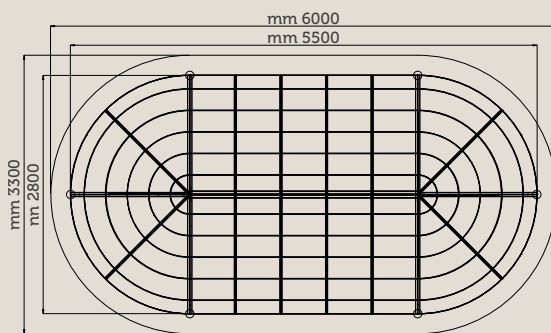
OV3360
