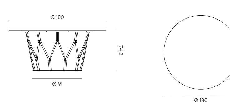
Tavolo da pranzo \varnothing 180 * Dining table \varnothing 180
