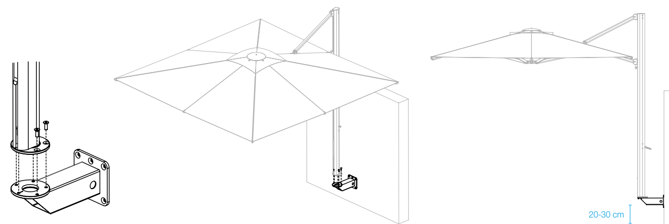
Cod. 1092 Fissaggio a muro—Cod. 1092 Wall console
