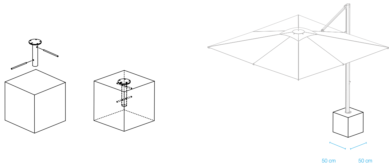
Cod. 1090 Fissaggio da cementazione—Cod. 1090 Submerged mounting plate
